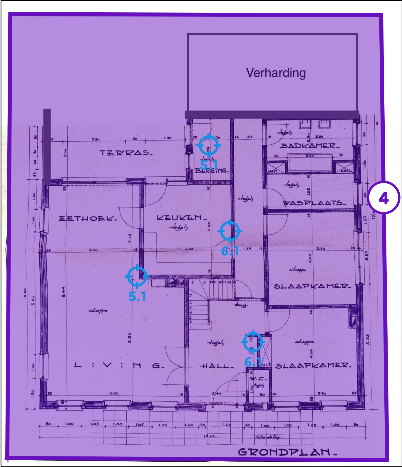
Legende van plan 1.2: Plan GLV Middenlaan 7 Leopoldsburg
